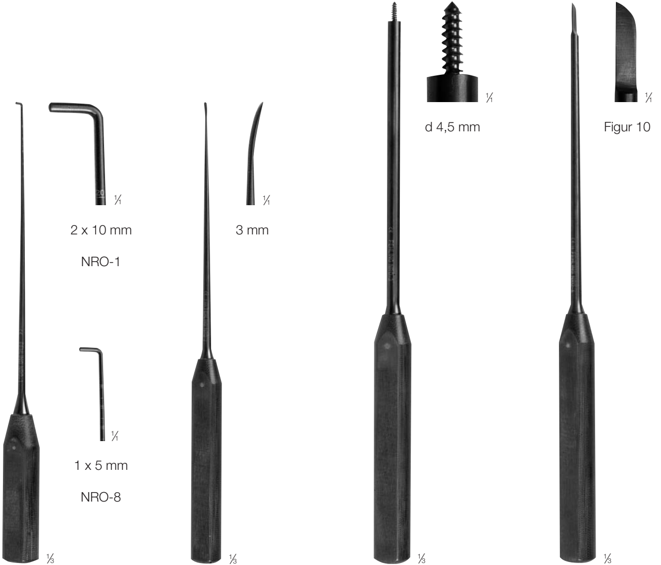
DISSECTOR, SEMI-SHARP DISSEKTOR, HALBSCHARF 370 mm
